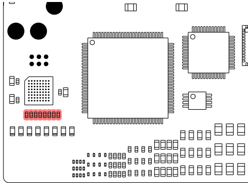
R105 R104 R106 R107 R108 R109 R110 8x 1k 0402-L Farnell 2447587
