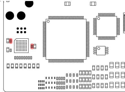
C10 C9 2x 100n 0402-L Farnell 1759380
