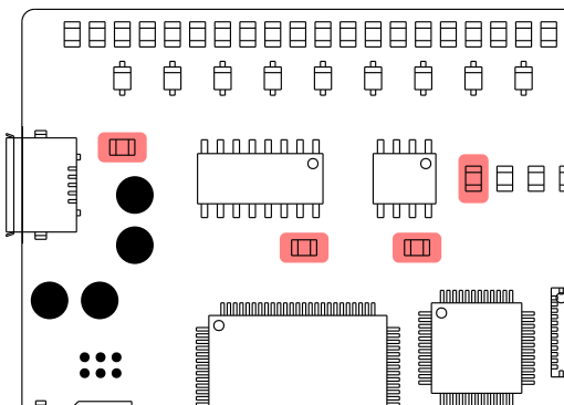
C3 C4 C1 C2 4x 100n 0805 Farnell 2496944
