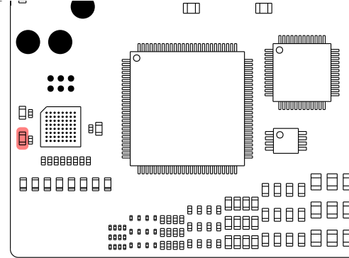
C8 1x 1μ 0603-L Farnell 2496916
