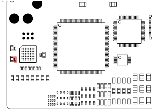
C11 1x 10n 0402-L Farnell 1758924
