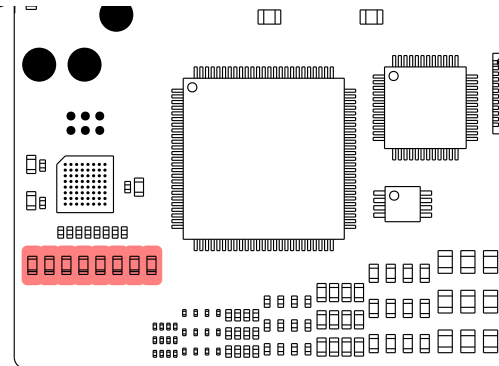
D23 D22 D24 D25 D26 D27 D28 D29 8x LED 0603-LED Farnell 2290329
